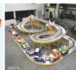
A0919 双环儿童爬山车 轨道高度1.9m高3.4m 规格: 1600x1000cm 12座 功率: 15kw 立方: 17m 3 电压: 380V 价格: 158000元 速度: 1.65m/s 轨道长度65m
